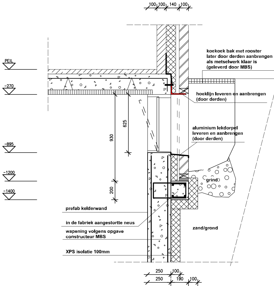
principe detail koekoek in kelderwand met neus
