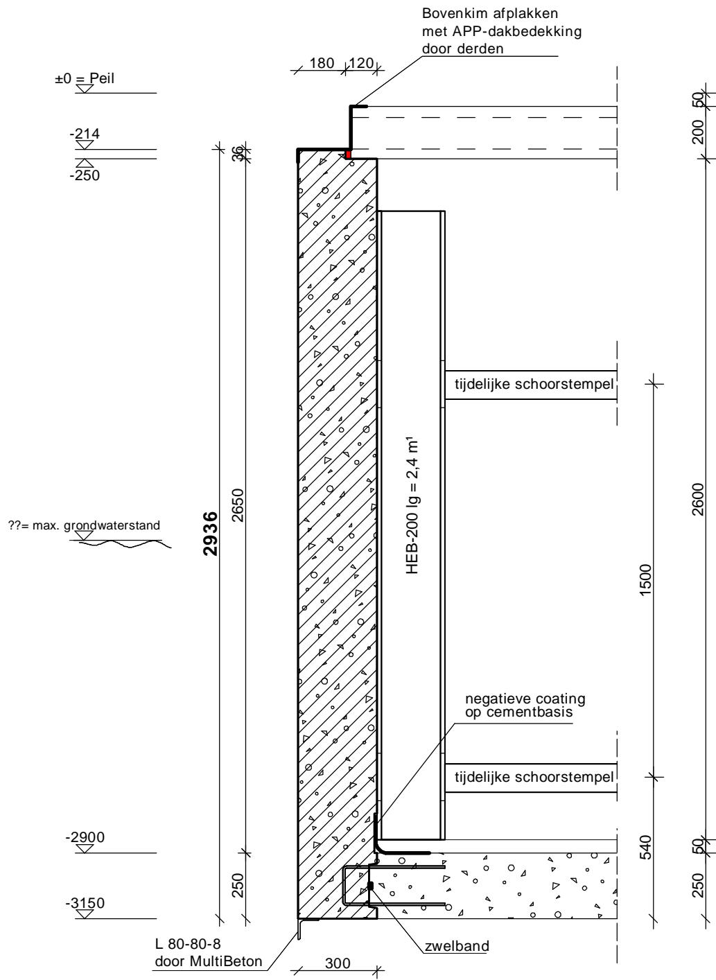
doorsnede A
